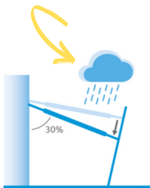
30 cm. hoogteverschil per 1 m. doeklengte
